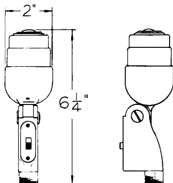
Fig. 4 — Dimensions
